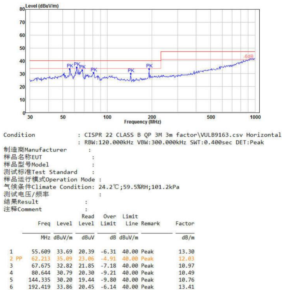
图 5-7 辐射测试垂直方向
