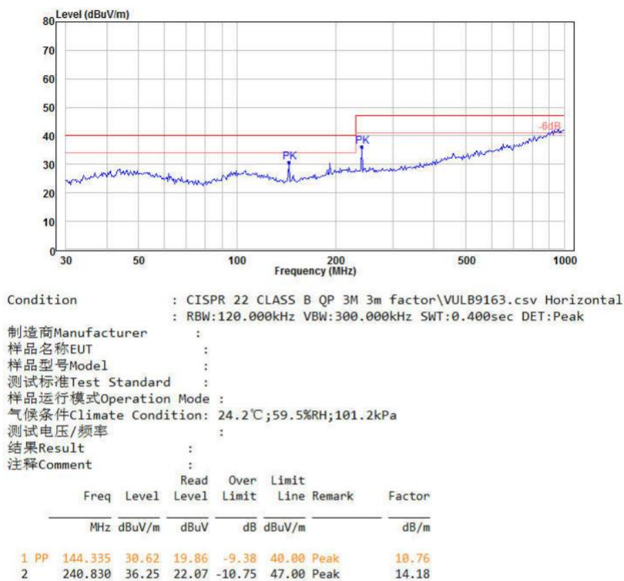
图 5-6 辐射测试水平方向
