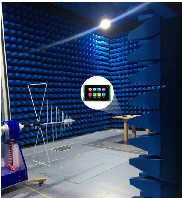
图 5-5 辐射测试图
