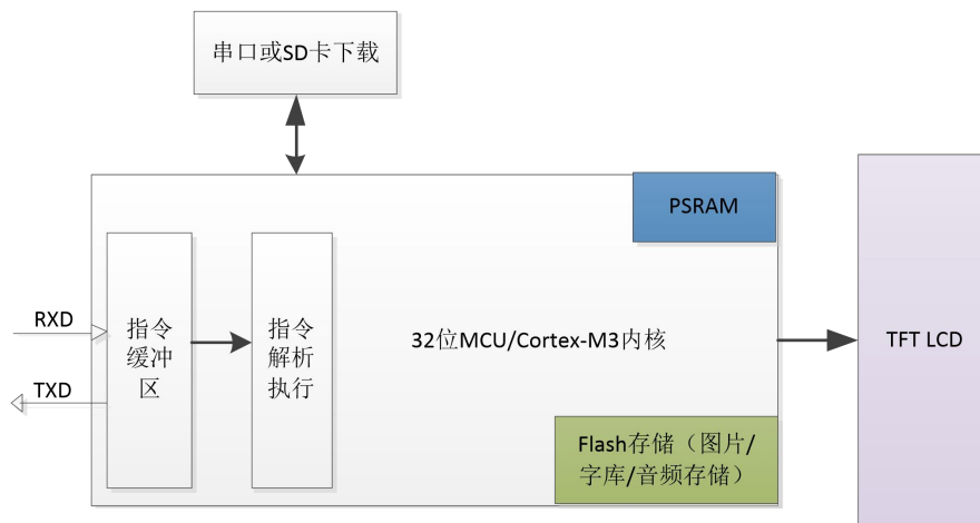
图 10-1 S 系列串口屏内部结构图
