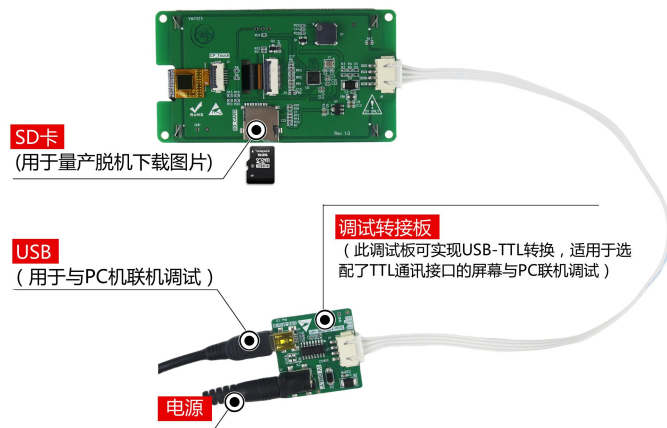
图 1-5 调试工具图
