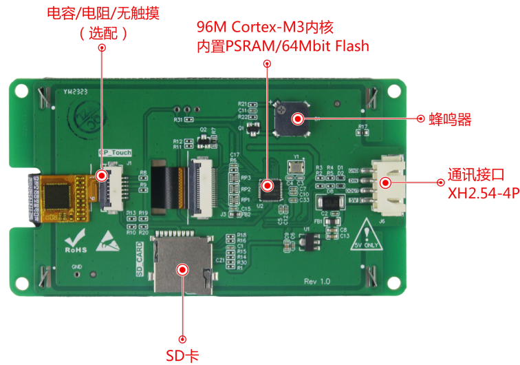
图 1-4 硬件配置图
